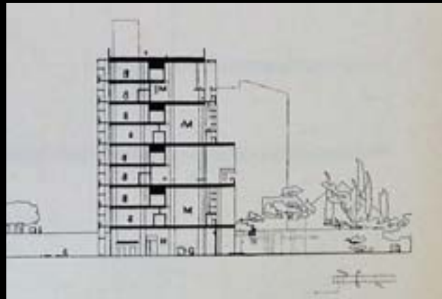
Secrétariat: coupe par la partie sur pilotis en double hauteur
