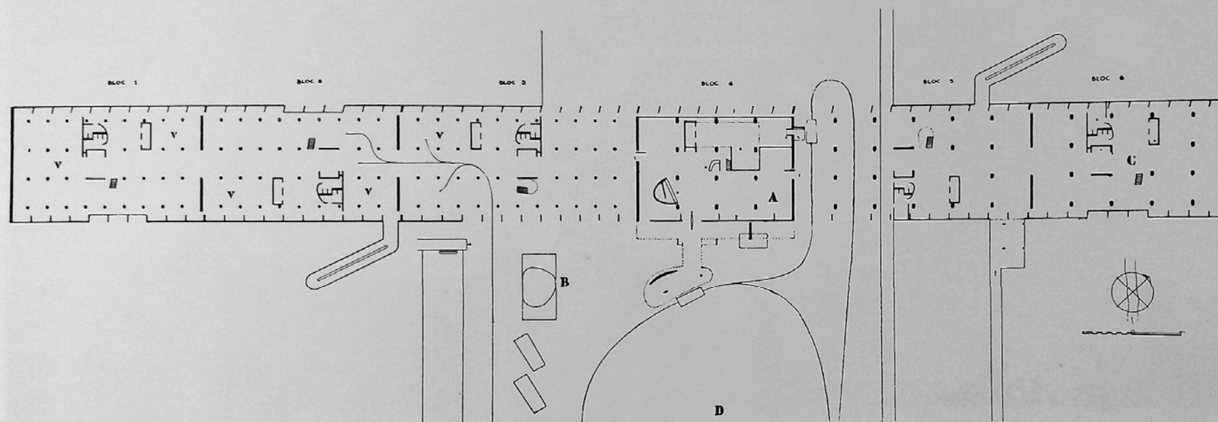
Plan des divers niveaux du Secrétariat
