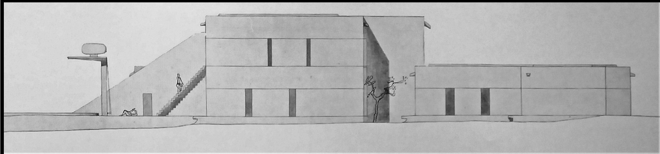
Elévation façade Est
